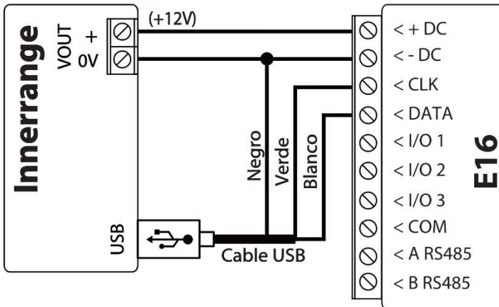
Diagrama de conexión de INNERRANGE INCEPTION con E16
